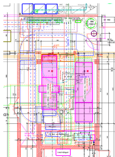
Lüftungszentrale
