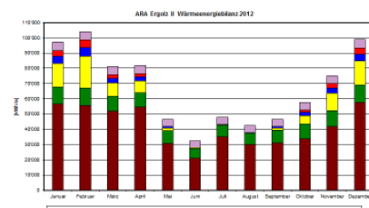
Wärmeenergiebilanz
